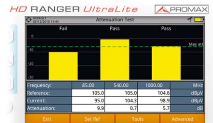
Attenuation test
